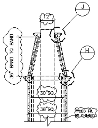
7 SECTION SCALE: 1/4" = 1'-0"
